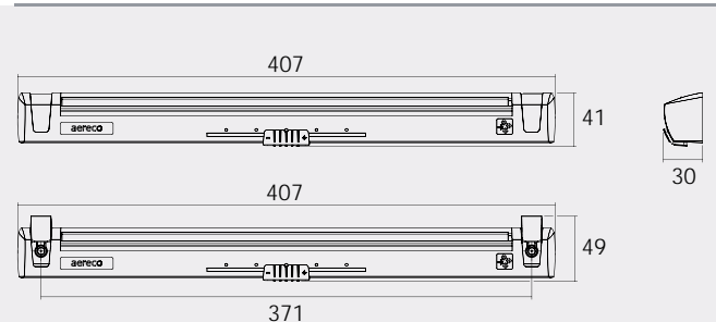
Méretek (mm) EFR típusú légbevezetők
